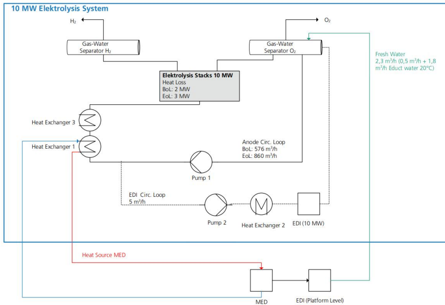
Abbildung 2-7: Blockschaltbild des 10-MW-Elektrolysesystems
