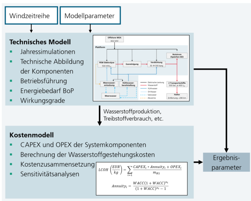
Abbildung 6-1: Schematischer Modellaufbau in H2ProSim im Offsh2ore Projekt
