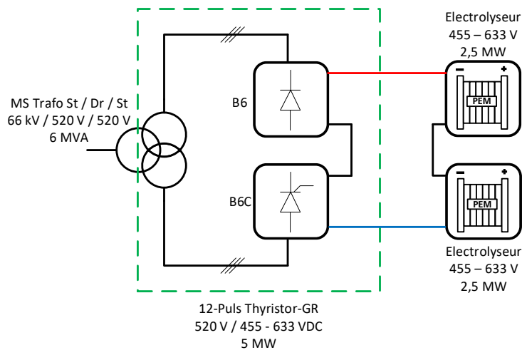
Abbildung 3-10: Anschlusschema des favorisierten Konzepts aus in Serie geschalteten Elektrolyseuren an einem 5 MW 12-Puls Thyristor-Gleichrichter mit Dreiwickler-Trafo
